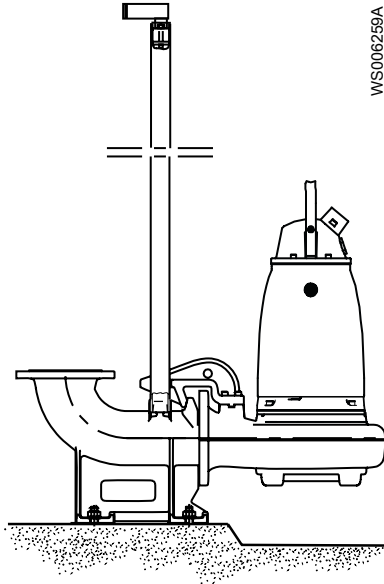
Рис. 2: Р-установка
